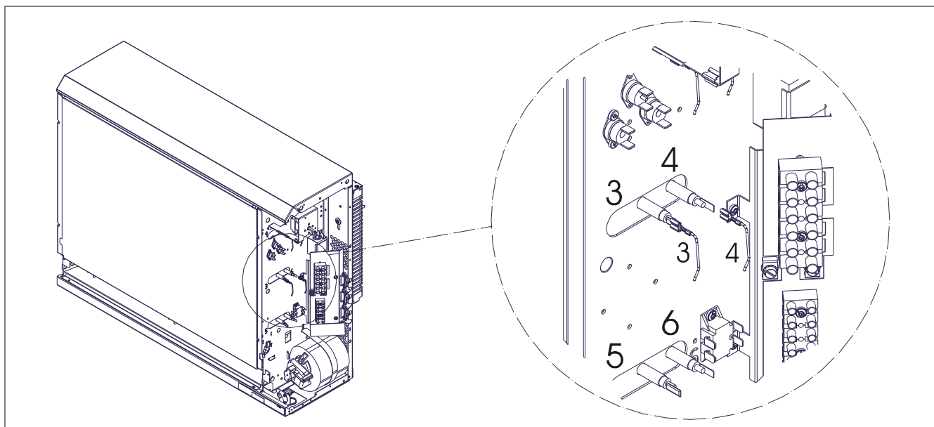
13. Na ścianie pośredniej oraz przewodach przyłączeniowych grzałek znajdują się numery (1-6). Przewody podłączyć do styków grzałek. Luźne przewody zamocować do wiązek.
