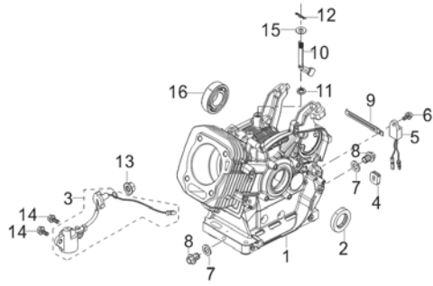
FIG.1 CRANKCASE. (E01)
