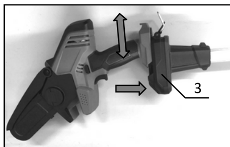
► 1. Connecting rod 2. Main tool body 3. Rod base
