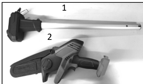
► 1. Connecting rod 2. Main tool body 3. Rod base
